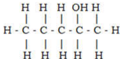
Pentan -2- ol
