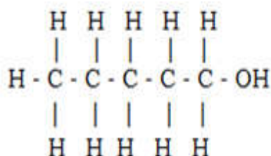
Pentan -1- ol
