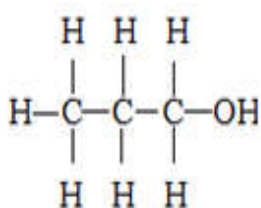
Propan -1- ol
