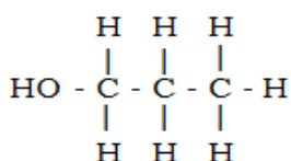
Propanol
