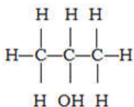
Propan -2- ol
